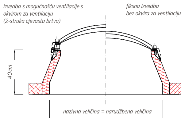
TOP-90 svjetlosna kupola na ISO-THERM nastavnom vijencu
